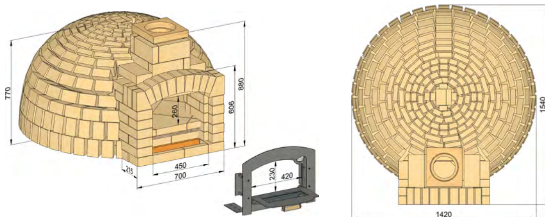
Pizzakuppel 110 Maße
